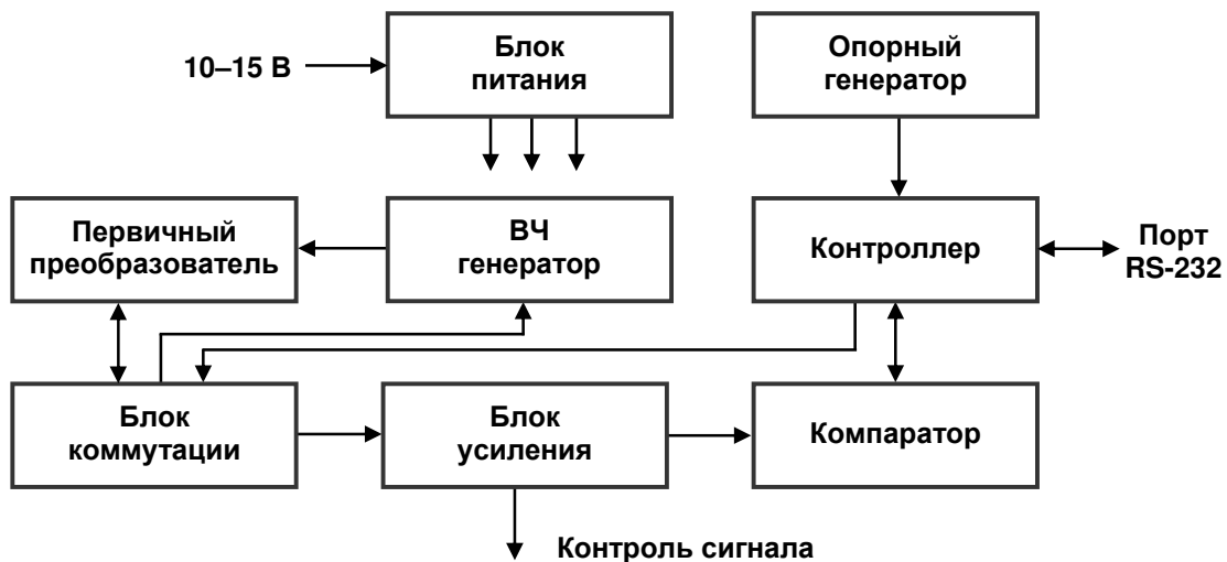
Рис. 1. Функциональная схема POS-1
